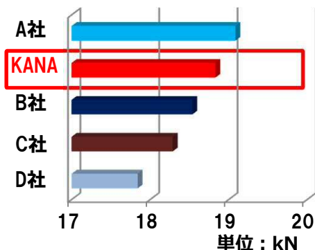
チェーン破断 実験データ
